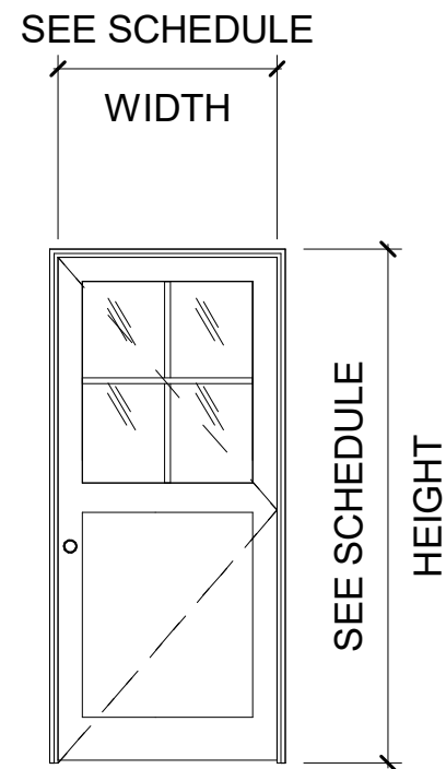
DOOR TYPE A3 - SGL SWING HALF LITE PANEL (DOORS 601.1, 602.2, 606.1)
