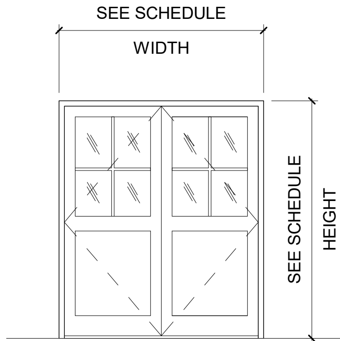
DOOR TYPE E1 - DBL SWING W/ HALF LITE (DOOR 603.1)
